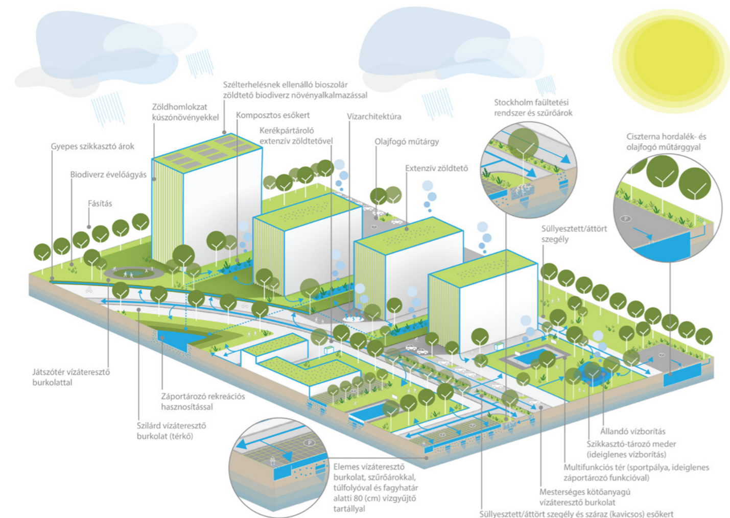
16. ábra Csapadékvíz helyben tartásának elősegítése teleszerű beépítés esetén
