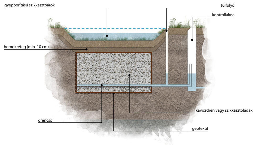
34. ábra Drénezett szikkasztóárok metszet
