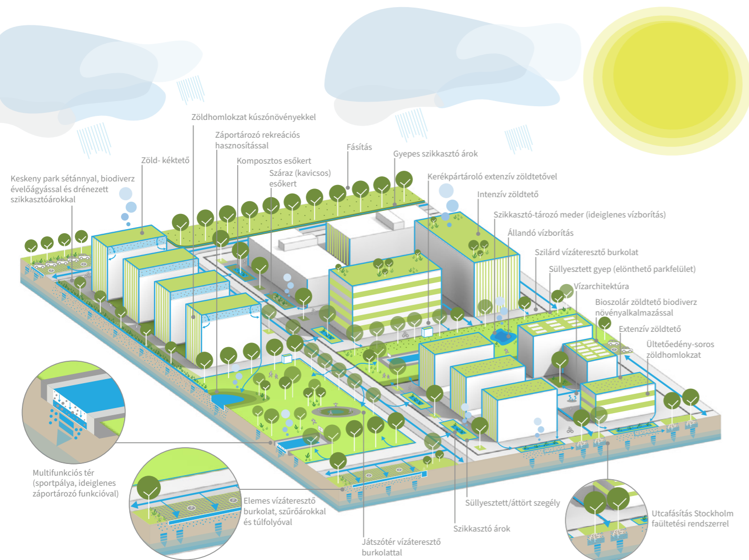
13. ábra Csapadékvíz helyben tartása komplex eszközök alkalmazásával új beépítések esetén
