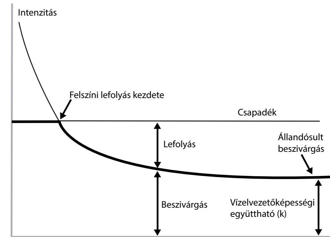
50. ábra Beszivárgási görbe
