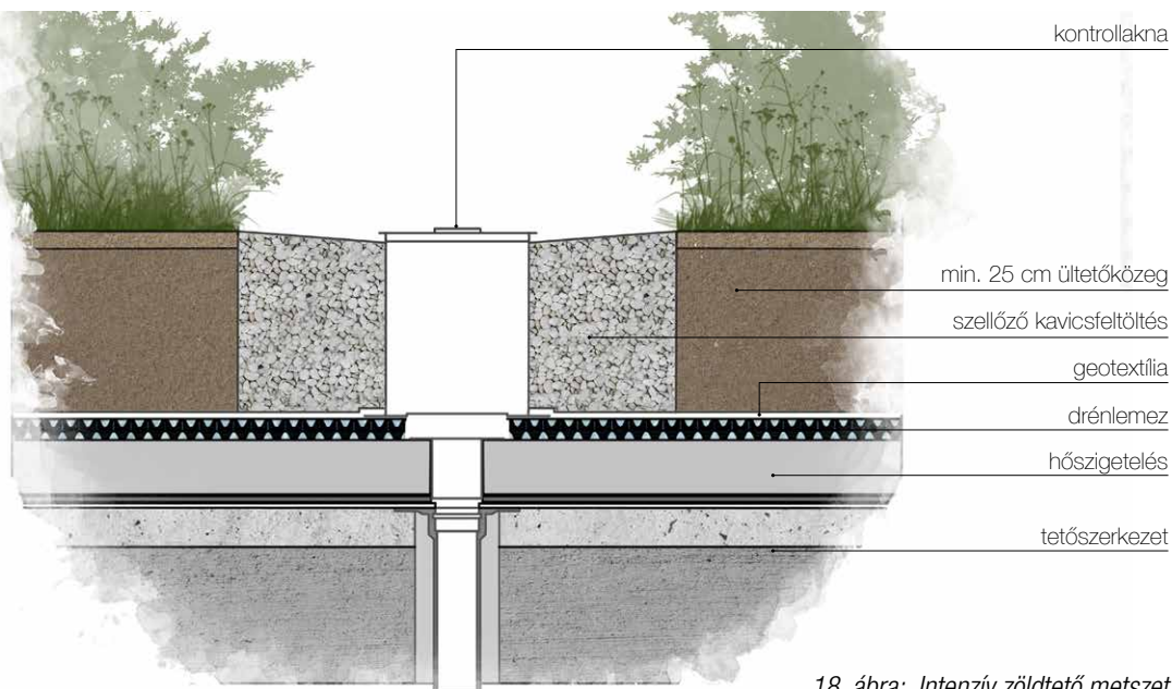
18. ábra: Intenzív zöldtető metszet
