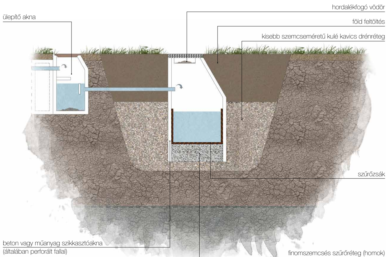
24. ábra: Dréncsőt ülepítőaknával
