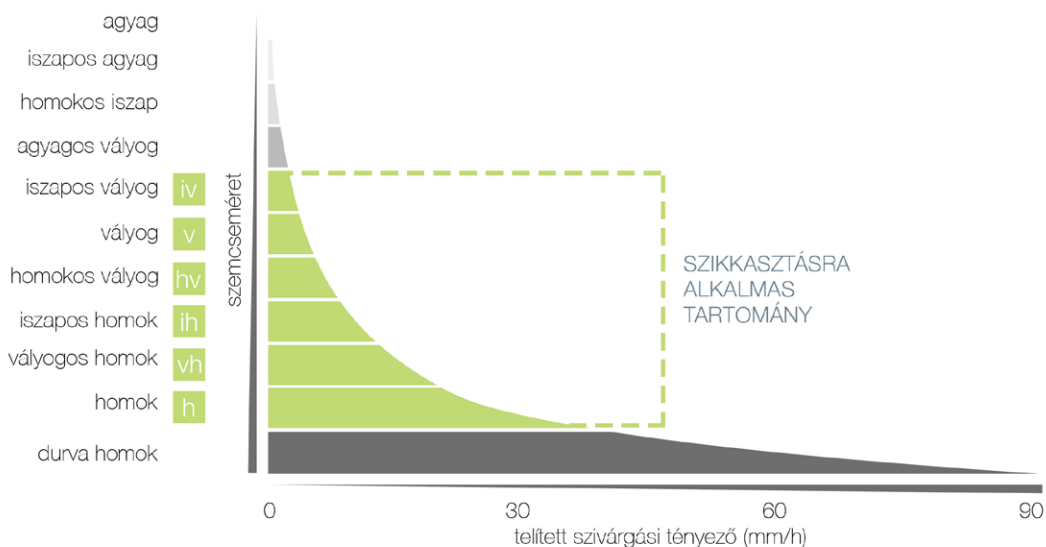
11. ábra: Talajtípusok vízáteresztő képessége (A. Makó, B. Debreczeni, Cs. Farkas, T. Hermann, P. Marth, F. Máté, 2011)
